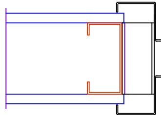
STEEL STUD ANCHOR
